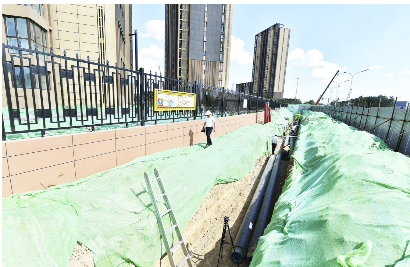
杨坨安置房供热管线工程施工现场,工人们正在焊接热力供热管网。记者 唐建/摄
